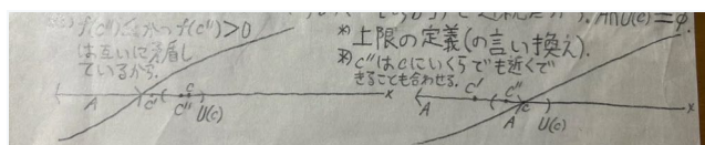
実軸の点の集合の右端が上限.
